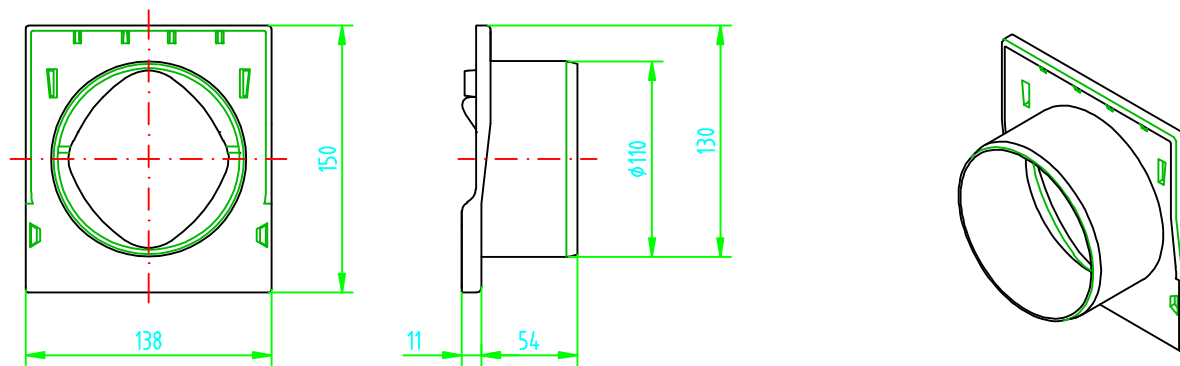
Čelní stěna pro konec žlabu s odtokem DN 100 - obj. č. 11087
