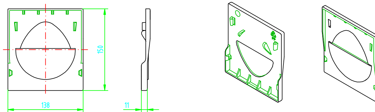
Kombinovaná čelní stěna pro začátek a konec žlabu - obj.č. 11086
